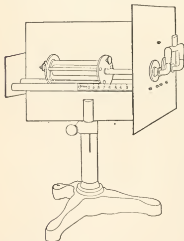
FIG. 19. Double Olfactometer (liquid stimuli).
